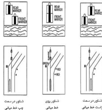
شکل ۳- استفاده از علائم چراغ هادی برای مکان‌یابی در کانال
