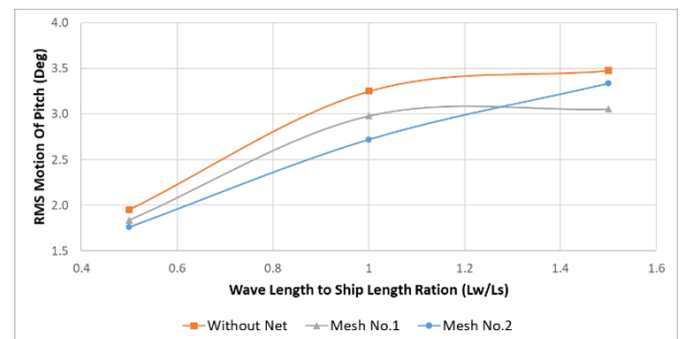
شکل ۱۷- مقایسه RMS حرکت پیچ مدل، مابین تور با مش ۱ و مش ۲ با بدنه بدون تور
