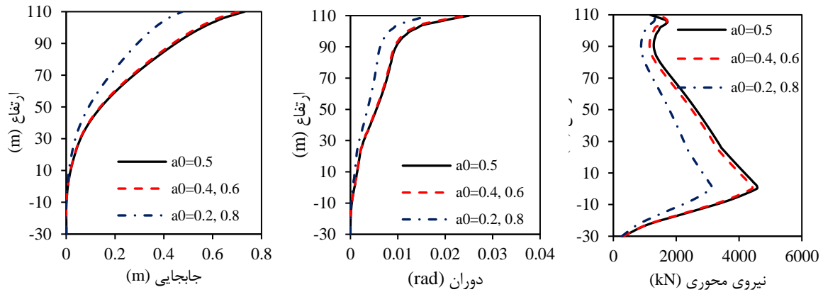
شکل ۹ - پاسخ‌هایی در طول برج و مونوپایل در معرض بار باد با فاکتور القایی متفاوت ( V_s = 11.4 m/s )
