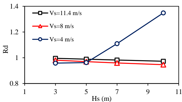
شکل ۱۱ - تأثیر ارتفاع موج بر پاسخ توربین بادی دریایی تحت ترکیب بار باد و موج ( T_s = 10Sec )
