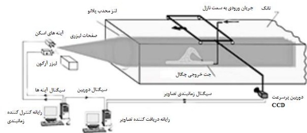
شکل ۱- نمای کلی از سامانه اسکن لیزری سه‌بعدی جهت آشکارسازی جریان آشفته به فلورسنت [۱۶]
