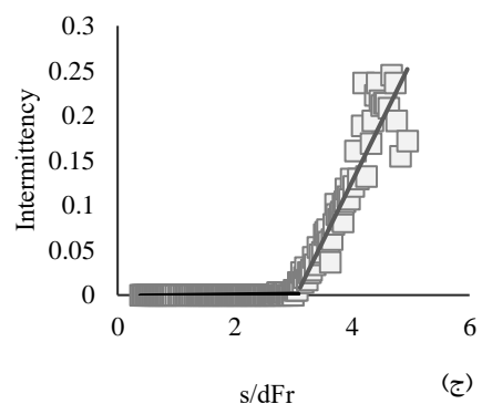
شکل ۷ - تغییرات در طول خط مسیر، (الف): ترقیق (ب): شدت آشفتگی (ج): تناوب
