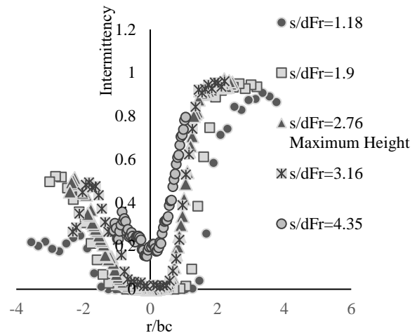
شکل ۶- تناوب در مقاطع عمود بر خط مسیر جریان در فواصل مختلف از منبع تخلیه
