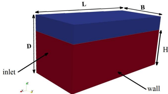
شکل ۲ - ابعاد دامن‌های حل و نوع شرایط مرزی اعمال شده
