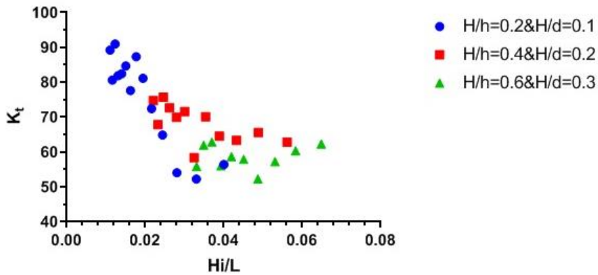
شکل ۱۴- ارائه‌ی نتایج ضریب عبور K_t در نسبت بی بُعد H/L برای مدل C
