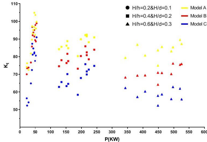
شکل ۲۰- مقایسه‌ی نتایج توانی سه مدل A، B و C
