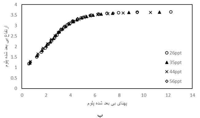
شکل ۸- نمیرخ پهنای بی بعد شده پلوم به ارتفاع بی بعد شده پلوم. نتایج روش عددی (الف) و روش آزمایشگاهی (ب)
