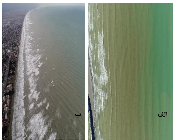
شکل ۲- نمونه ای از تصاویر برداشت شده توسط پهپاد -مقدار عرض شکست با استفاده از خط کش گوگل ارث در تصویر الف ۶۷ متر و در تصویر ب ۱۰۵ متر است. تصویر ب وضعیت منطقه شکنا در زمان وقوع بیشترین عرض شکست را طی دوره مطالعاتی نشان می دهد.
