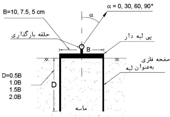
شکل ۳- جزئیات مدل‌های پی لبه‌دار مورد استفاده در آزمایش‌ها
