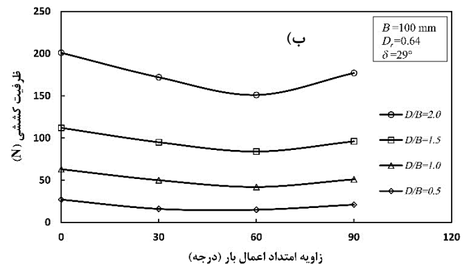
شکل ۱۱- تغییرات ظرفیت کششی مدل‌های پی لبه‌دار به‌ازای زوایای اعمال بارگذاری؛ الف) منحنی بار-جاب‌جایی، ب) مقادیر ظرفیت کششی برحسب زوایای اعمال بارگذاری
