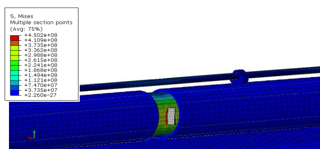
شکل ۲۱- تنش وارده به خط لوله در اثر اعمال نیروی ۶۰ تن
