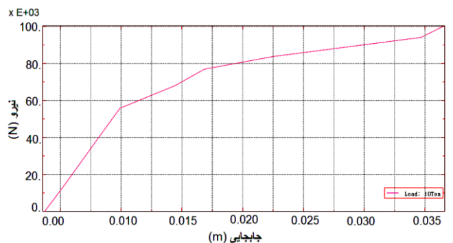
شکل ۱۶- نمودار نیرو - جابجایی در اثر اعمال نیروی ۲ تن
