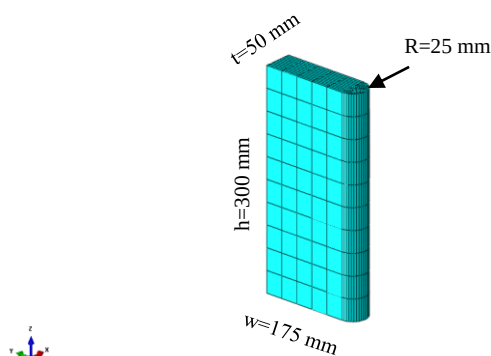
شکل ۱۱- مدل سنبه مطابق با آئین نامه DNV-RP F-111
