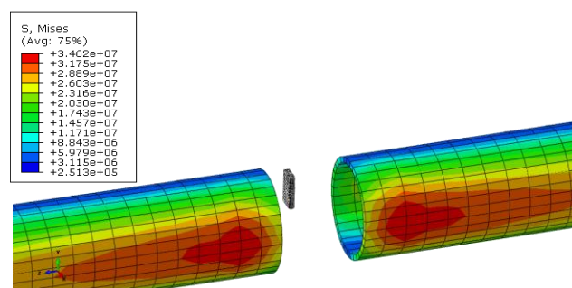
شکل ۲۳- تنش وارده به به عایق بتن در اثر اعمال نیروی ۶۰ تن
