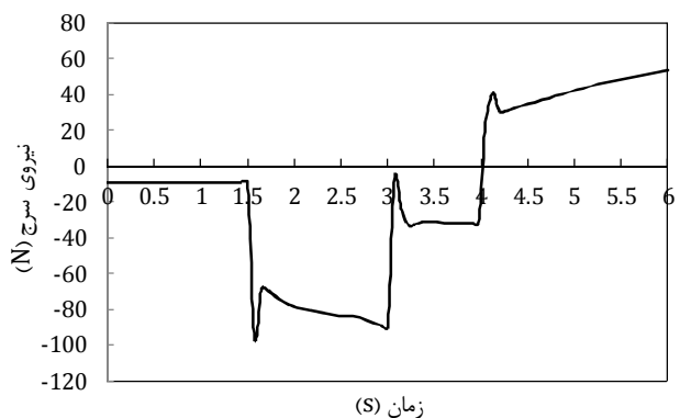
شکل ۱۶- نمودار تغییرات نیروی سرچ در حرکت شتابدار سرچ
