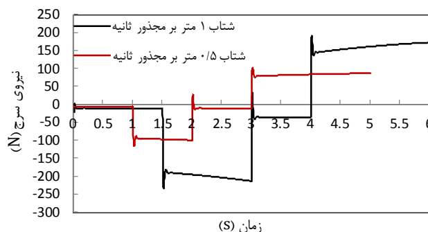
شکل ۱۱- نمودار تغییرات نیروی وارد بر بیضیگون در راستای طولی در دو حرکت با شتاب های متفاوت
