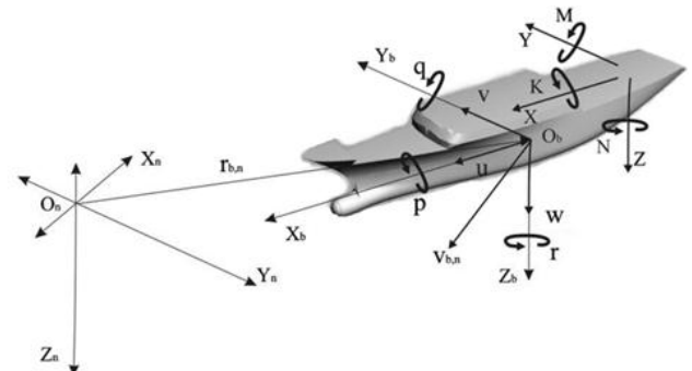
شکل ۱- مختصات ثابت و متحرک در حرکت شناور [۱۷]
