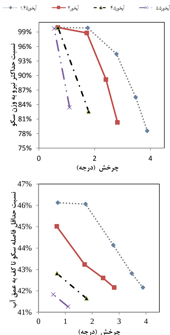
شکل ۱- تاثیر پارامتر میزان چرخش اولیه بارج بر حداقل فاصله تا کف (نمودار پایینی) و حداکثر نیروی وارد شده بر سکو در حین آب اندازی (نمودار بالایی) - سکوی ۸ پایه
