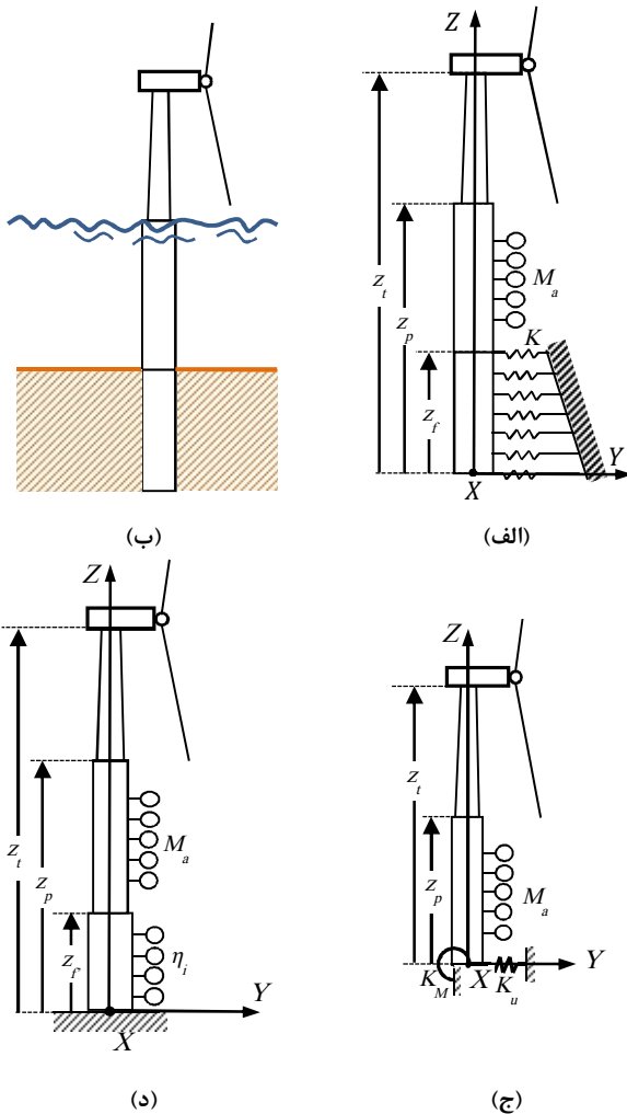
شکل ۲- الف) مدل DS، ب) توربین بادی فراساحلی با سکو تک شمع، ج) مدل CS، د) مدل AF
