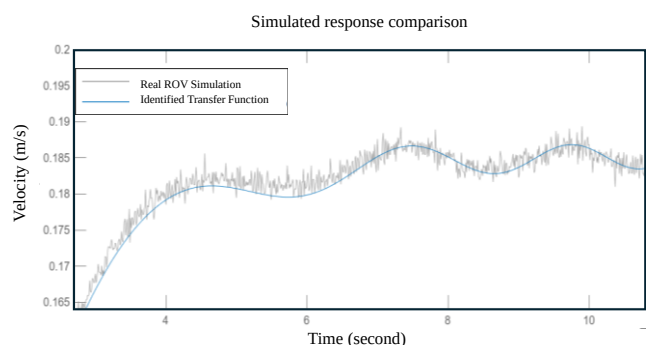
شکل ۱۸- برازش تابع تبدیل بر مدل با نویز خروجی
