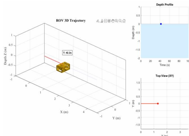
شکل ۷- شبیه‌سازی و صحت‌سنجی در حرکت سرج
