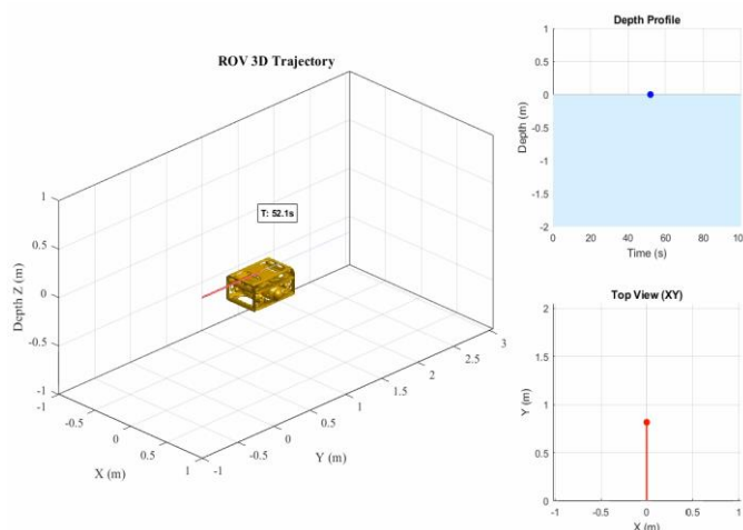
شکل ۸- شبیه‌سازی و صحت‌سنجی در حرکت سوی
