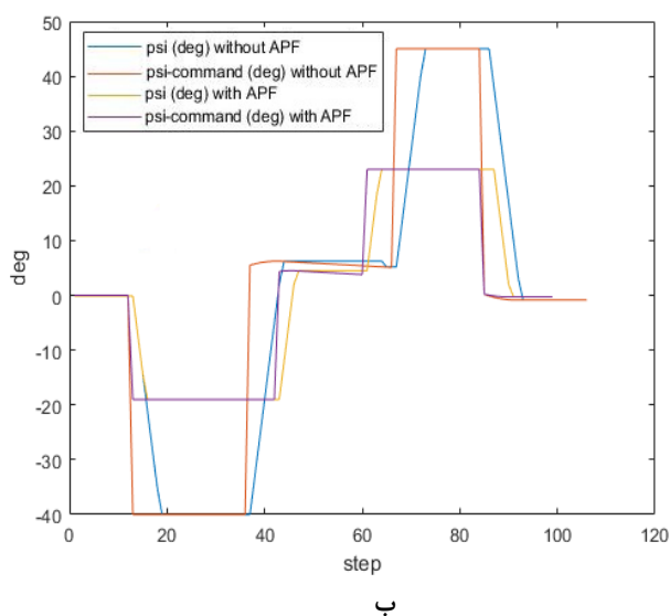
شکل ۲۳- الف) مقایسه مسیر فرار از موانع، ب) مقایسه زاویه فرمان سمت
