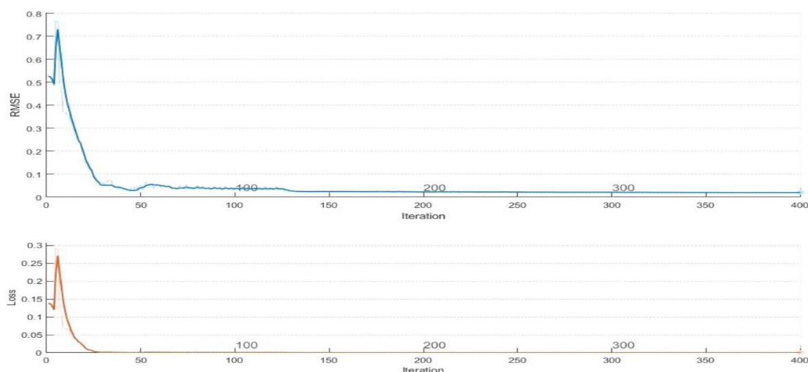
شکل ۱۷- نمودار RMSE و اتلاف برای آموزش شبکه LSTM جهت تخمین حرکت موانع
