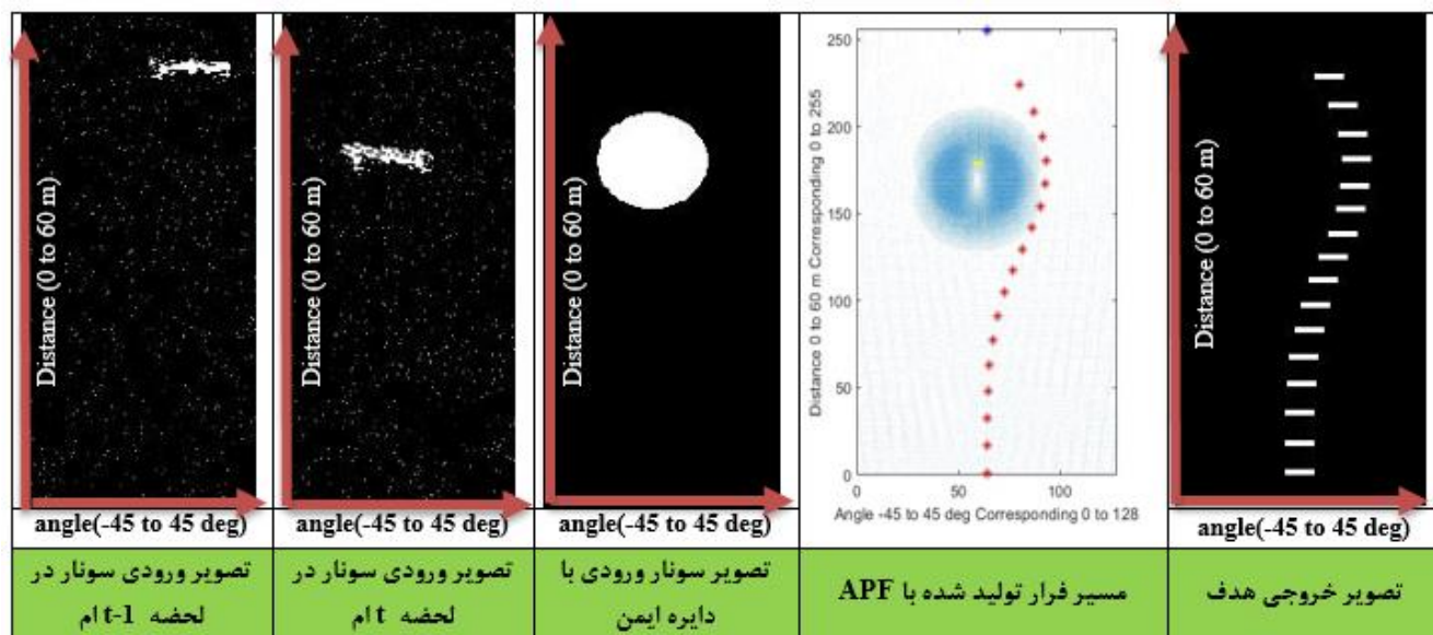
شکل ۱۰- نمونه ای از تصویر ورودی سونار و تصویر منطقه امن متناظر آن، به همراه تصویر مسیر فرار بدست آمده از روش پتانسیل مجازی و تصویر هدف شبکه جهت آموزش، بدست آمده از روش SFM
