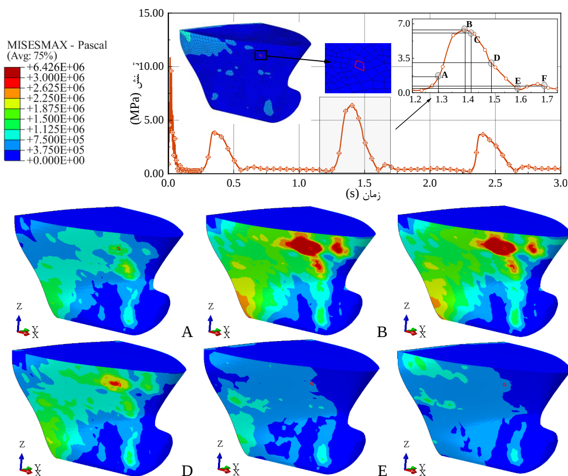
شکل ۲۱- تغییرات تنش معادل بر روی پوسته بیرونی ناحیه سینه کشتی در بازه دومین کوبش به سطح آب بر روی یک جزء.
