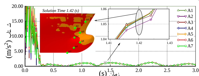
شکل ۲۳- نمودار شتاب ناشی از کوبش در هفت نقطه مشخص شده
