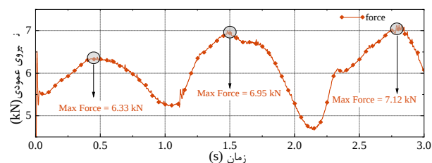
(ب) نیروی عمودی
