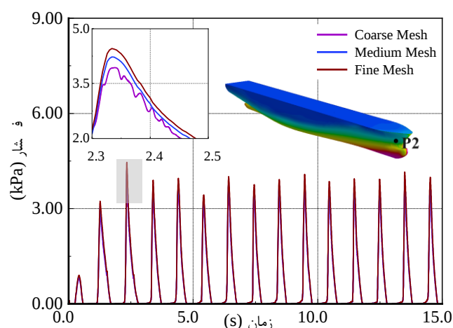
الف) فشار ناشی از کوبش در ناحیه پهلوی - نقطه ۲
