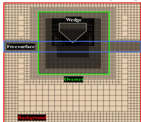
شکل ۱۰- جزئیات طرح شبکه بندی گوه.
