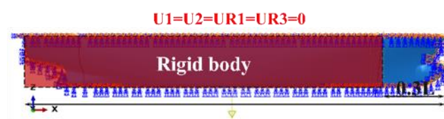
شکل ۷- شرایط مرزی اعمال شده در آباکوس.
