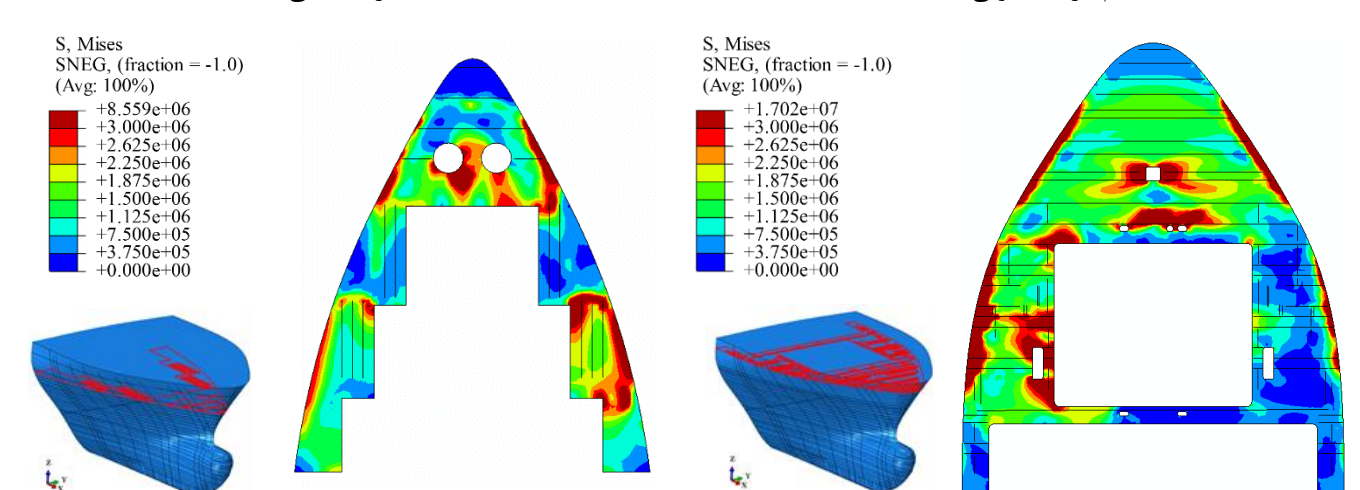
عرشه اصلی
