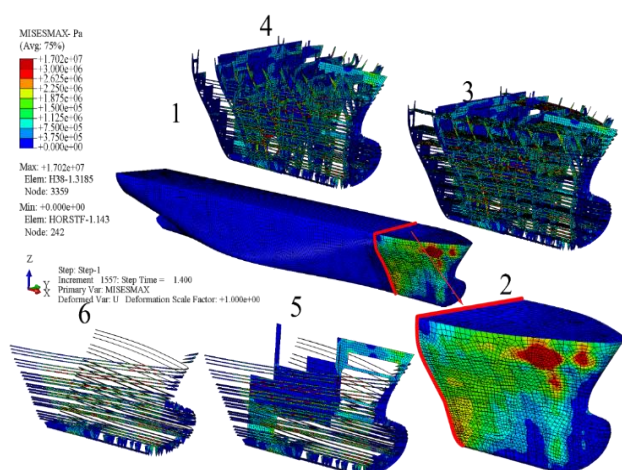
شکل (۱۸): توزیع تنش معادل بر سازه سینه کشتی.
