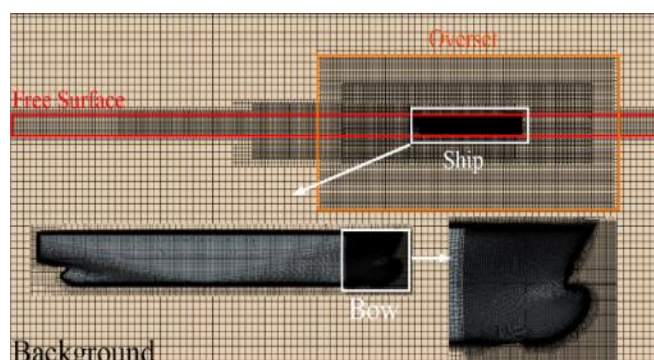
شکل ۱۲- جزئیات شبکه بندی در اندازه شبکه ی ریز.
