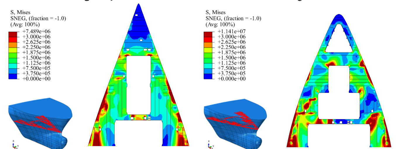
عرشه میانی
