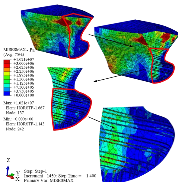
شکل ۲۰- توزیع تنش معادل در تقویت‌کننده‌های بدنه کشتی.
