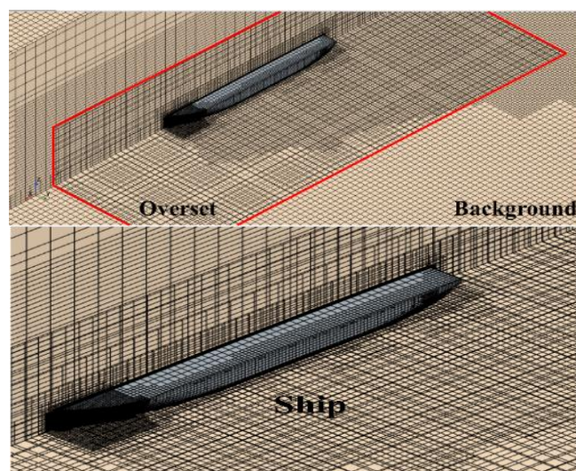
شکل ۴: طرح شبکه‌بندی در دینامیک سیالات محاسباتی.
