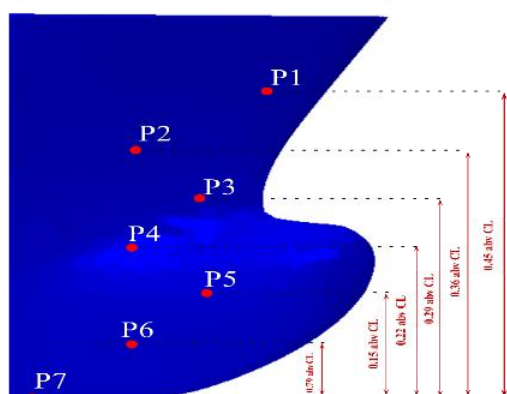
شکل ۵- نقاط تعیین شده بر روی سینه کشتی.
