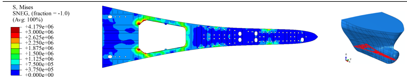
عرشه میانی
