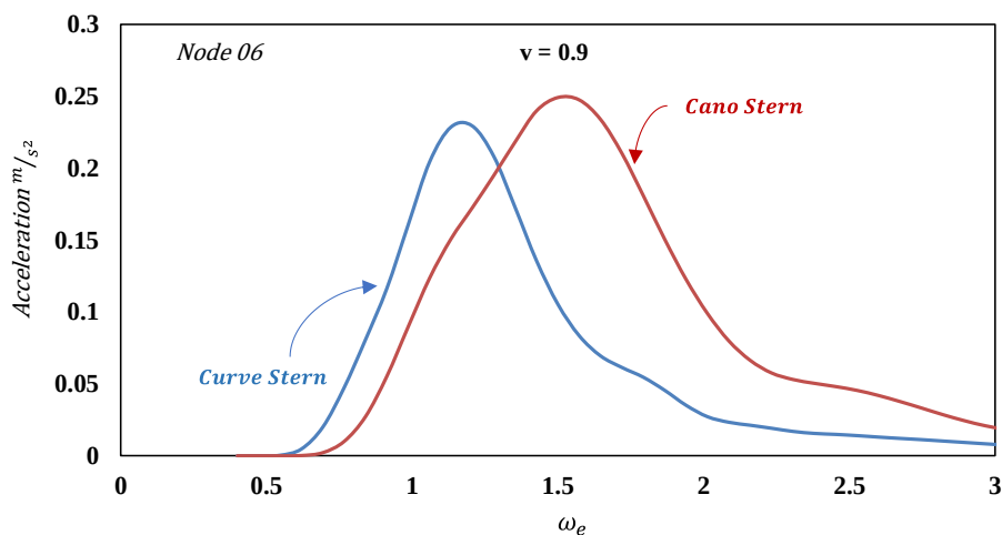
شکل ۱۴- نمودار شتاب برای هر دو فرم پاشنه در سرعت ۱۰ نات و نقطه ۶
