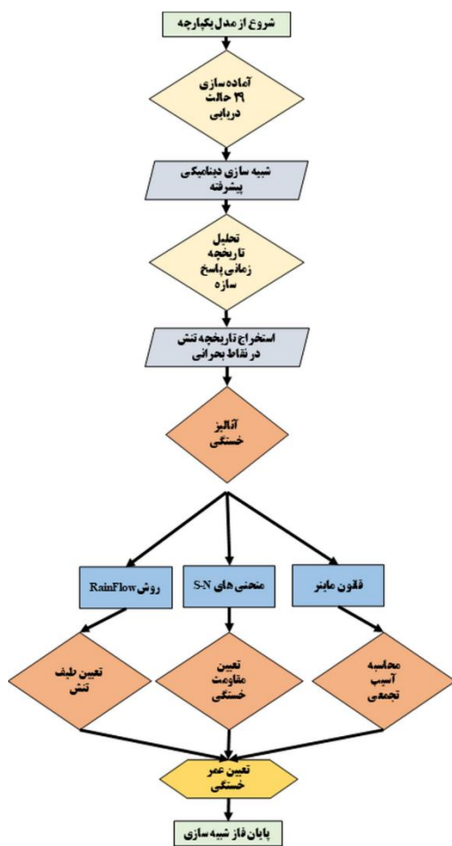
شکل ۴- روندنمای فاز شبه‌سازی و تحلیل دینامیکی
