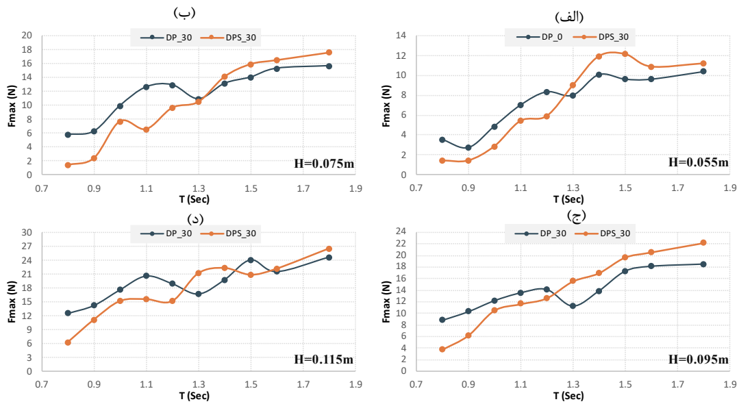
شکل ۷- مقایسه بیشینه نیرو وارد به مهار جلو سازه بین سازه DP_30 و DPS_30 بر حسب پریود در ارتفاع امواج مختلف (الف): H=0.055m (ب): H=0.075m (ج): H=0.095m (د): H=0.115m
