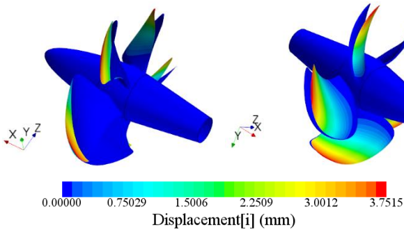
شکل ۳۵: کانتور جابه‌جایی x در J=1.2 ، E=0.7 GPa و \nu = 0.33
