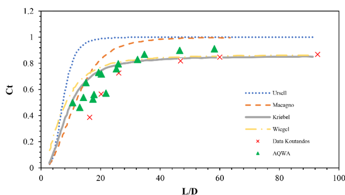
شکل ۳- داده‌های آزمایشگاهی Koutandos و همکاران (۲۰۰۵) برای موج‌شکن ثابت در مقیاسه با مدل عددی AQWA، امواج منظم ( H=2m ) [۲۱-۲۴] ( B=2m )
