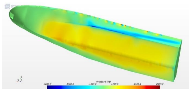
شکل ۱۳- توزیع فشار در عدد فرود ۱/۱۹ در یکی از زوایای دریفت
