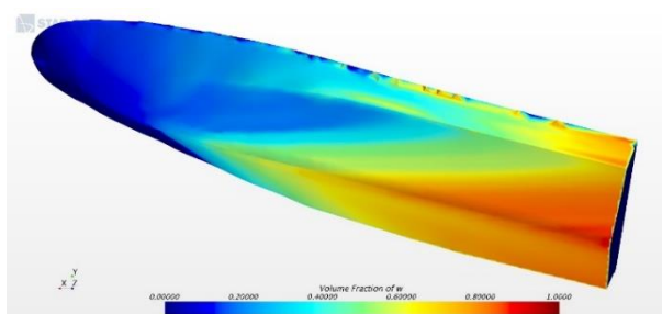
شکل ۱۲- سطح خیس در زوایای دریفت مختلف در عدد فرود ۱/۱۹
