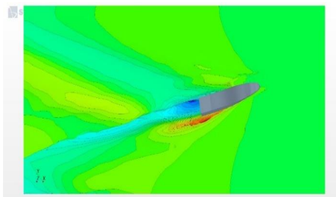
شکل ۱۱- نمونه‌ای از الگوی موج کلون در یک زاویه دریفت
