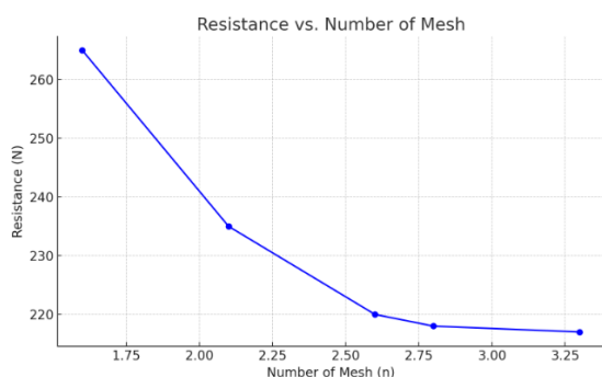
شکل ۸- مقایسه مقاومت شناور ناجی در مش بندی های مختلف
