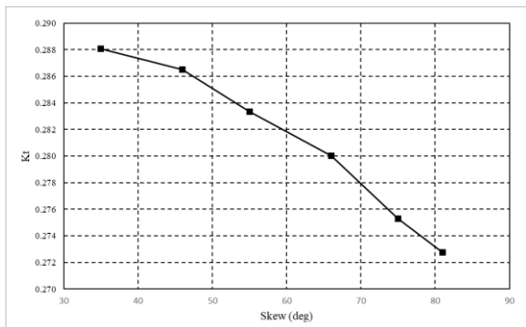
شکل ۱۴ نمودار ضریب گشتاور در سرعت دورانی ۳۰۰۰ دور بر دقیقه و
