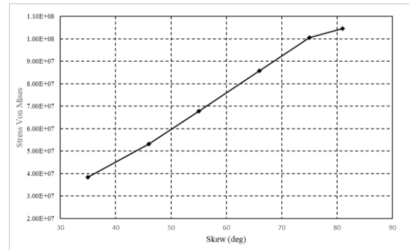
شکل ۱۶ نمودار تنش بیشینه در سرعت دورانی ۳۰۰۰ دور بر دقیقه و ضریب پیشروی ۰/۴ برای پروانه با اسکيو متفاوت
