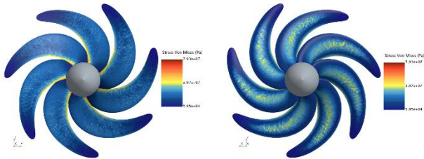
زاویه اسکيو ۸۱ درجه
