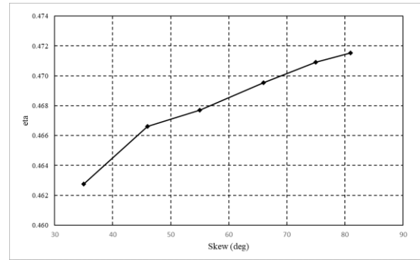
شکل ۱۵ نمودار بازده در سرعت دورانی ۳۰۰۰ دور بر دقیقه و ضریب پیشروی ۰/۴ برای پروانه با اسکيو متفاوت
