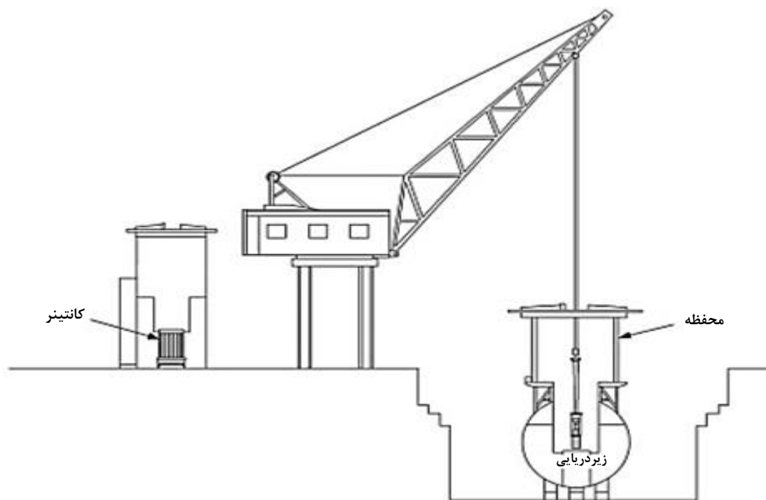
شکل ۲- سوخت‌گیری زیردریایی [۲]
