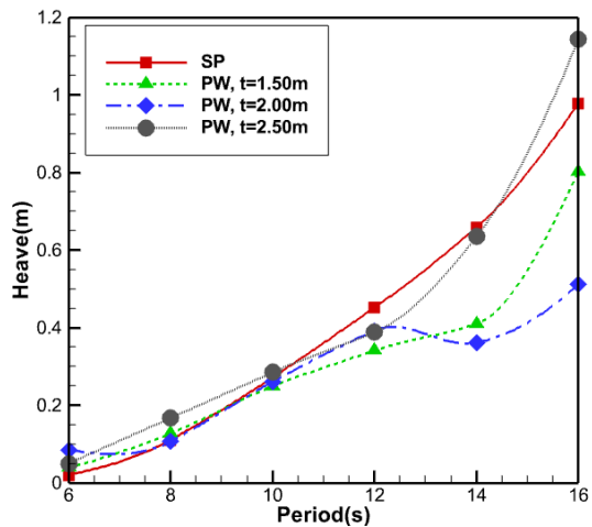
شکل ۱۶- تاثیر ضخامت فلپ روی دامنه هیو سکوی ترکیبی و سکوی تنها
