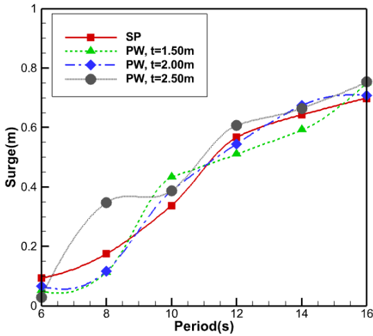
شکل ۱۴- تاثیر پهناي فلپ روی دامنه جابجایی فلپها تنها
