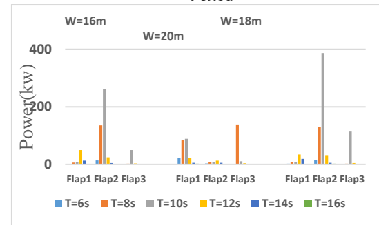
شکل ۱۵- تاثیر پهناي فلپ روی توان تولیدی مبدل های انرژی
