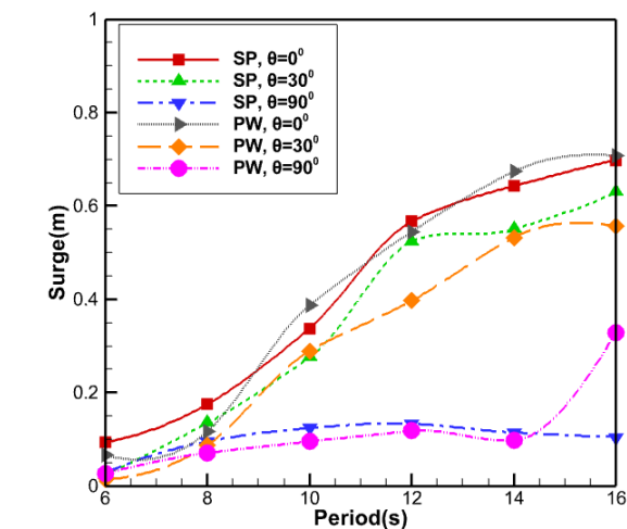
شکل ۲۲- تاثیر زاویه برخورد موج روی دامنه سرچ سکوی ترکیبی و سکوی تنها
