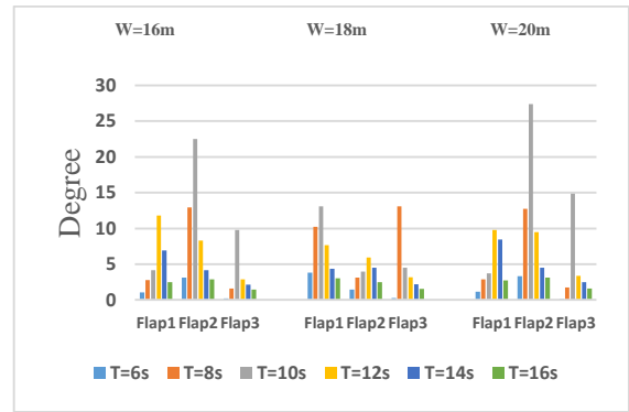
شکل ۱۴- تاثیر پهناي فلپ روی دامنه جابجایی فلپها
