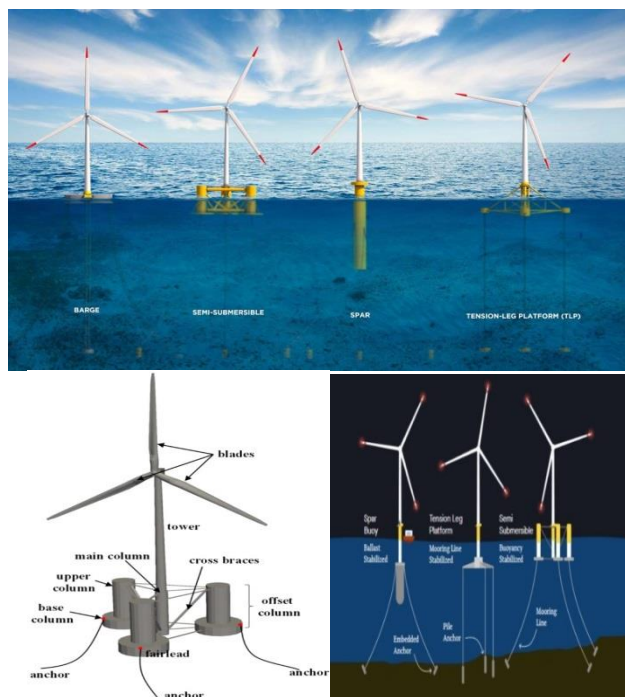
شکل ۱- انواع توربین بادی شناور دور از ساحل [1,2]
