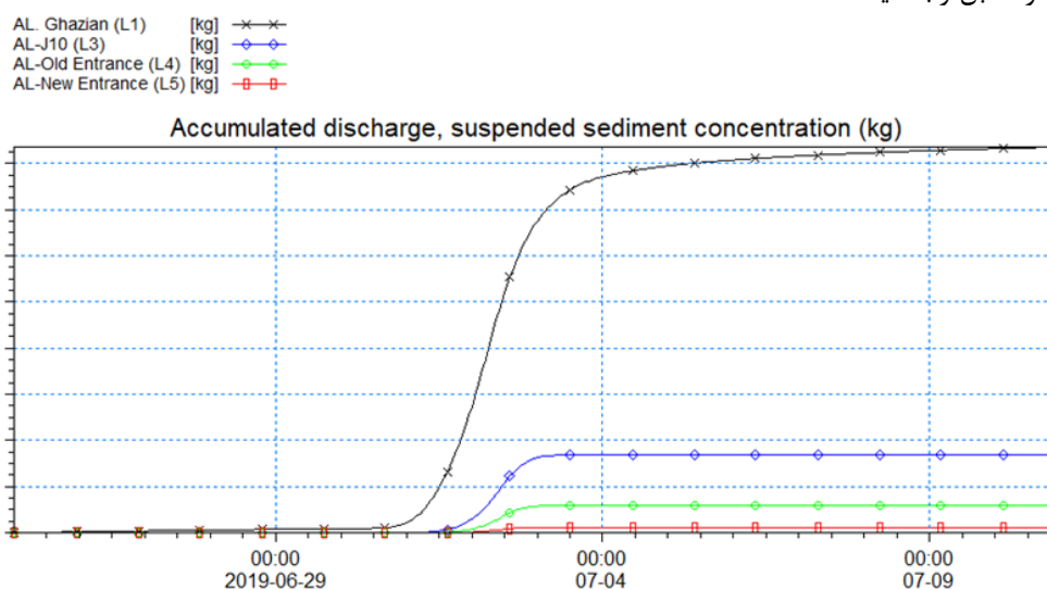
شکل ۱۳- مقادیر تجمعی عبور رسوبات از مقاطع کنترل در سیلاب ضعیف
