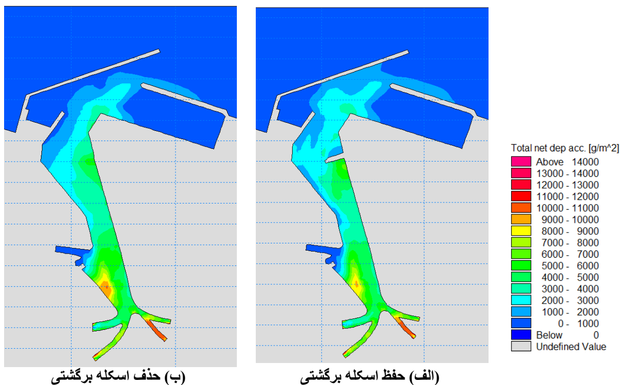
شکل ۱۴- الگوی نشست رسوبات در محدوده بندر در طول سیلاب متوسط
