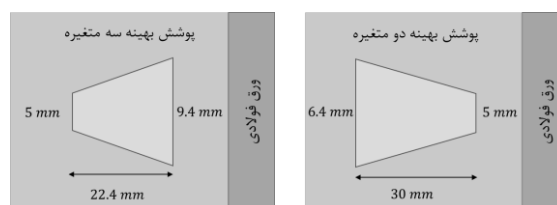
شکل ۲۷: شکل هندسی حفره پوشش‌های بهینه بدست آمده در دو حالت دو و سه متغیره
