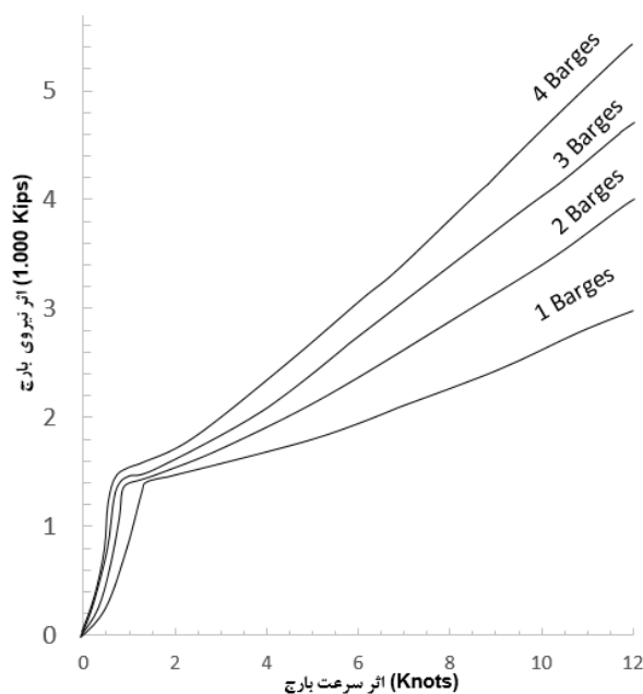
شکل ۳: اثر نیروی ناشی از برخورد بارج متناسب با سرعت شناور [۱۲]
