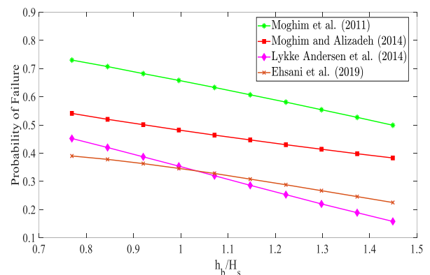
شکل ۱۴- تأثیر پارامتر بدون بعد h_b بر احتمال خرابی سکوی موج‌شکن در مدل‌های مقیم و همکاران (۲۰۱۱)، مقیم و علیزاده (۲۰۱۴)، لیک اندرسن و همکاران (۲۰۱۴) و احسانی و همکاران (۲۰۲۰) در مقطعی با تراز کف ۱۳/۸-
