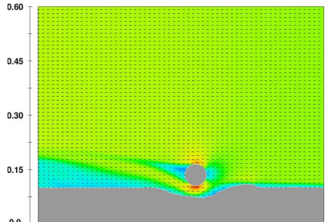
شکل ۹- پروفیل آبشستگی برای t=800 s (سیکل اول)
