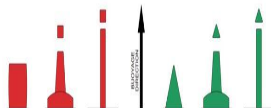
شکل ۴- بویه علائم جانبی
