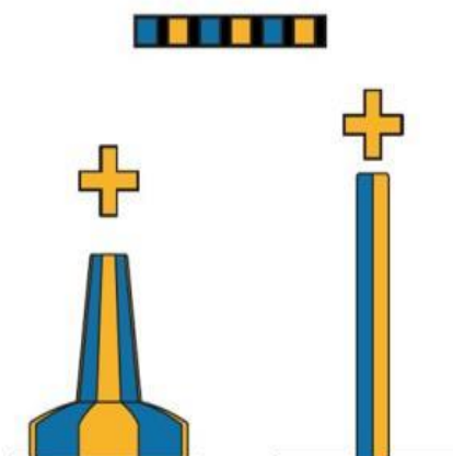
شکل ۹- بویه‌های خطر جدید
