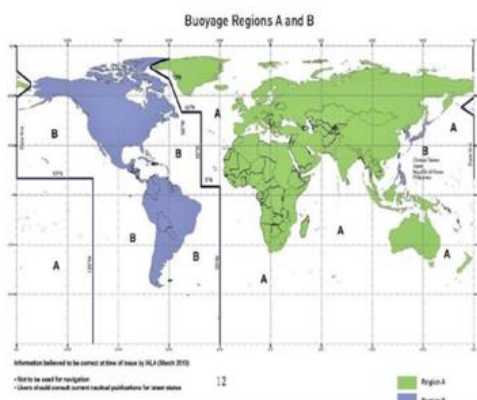
شکل ۴- مناطق A و B با قرارداد بویه گذاری A و B
