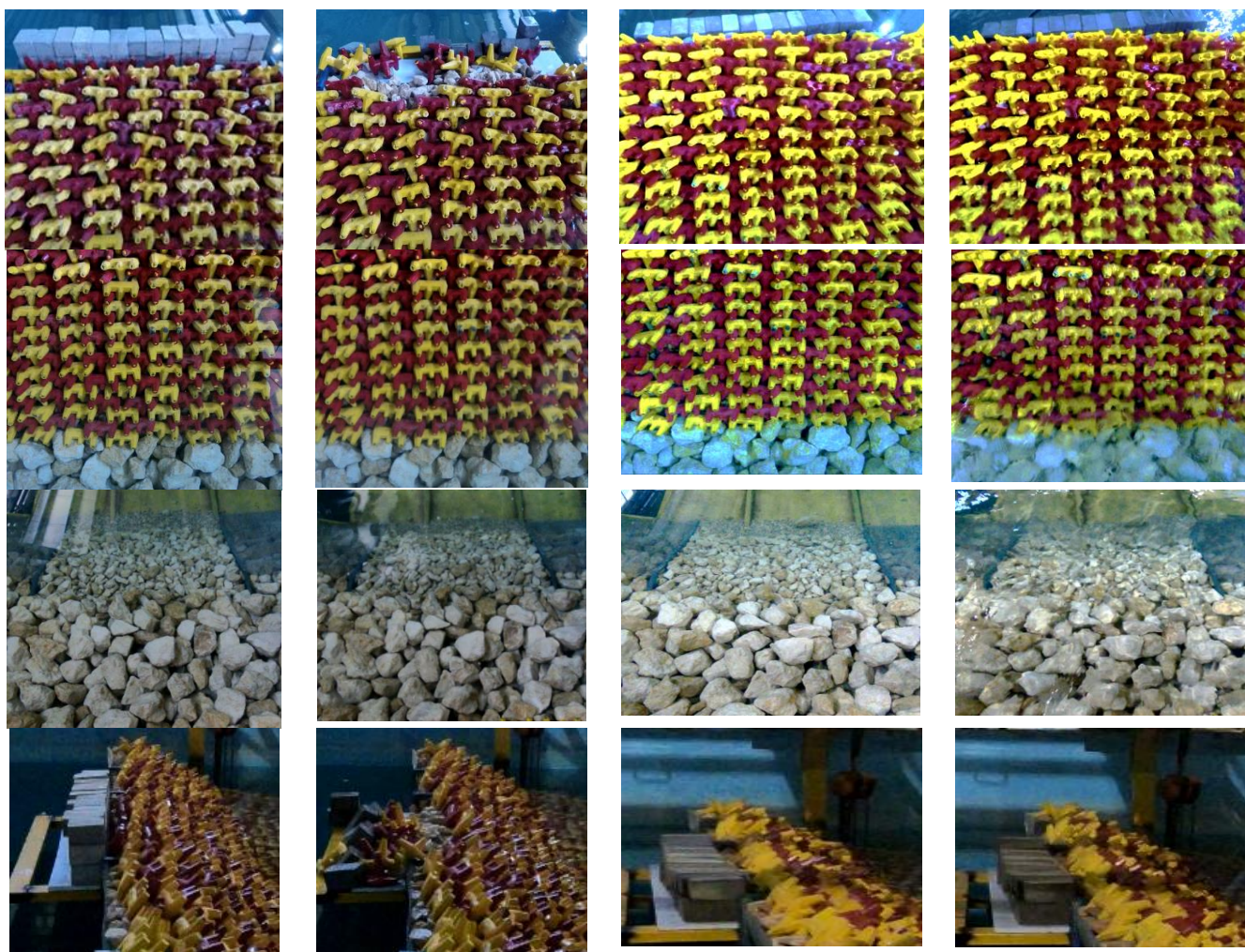
آزمایش شماره ۱ ( T_p=2.23 , H_s=28 , d=108 )
