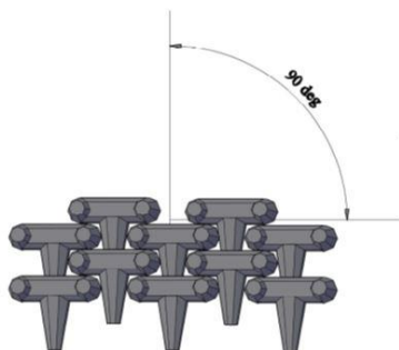
شکل ۶- نحوه قرارگیری آرمور جدید به صورت یک لایه با زاویه ۹۰ درجه
