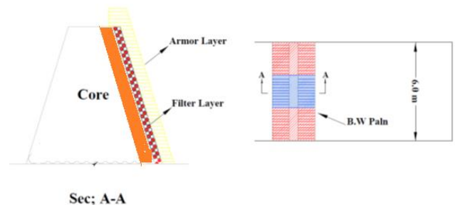
شکل ۵- پلان و نحوه چینش مصالح آرمور، فیلتر و هسته در فلوم آزمایشگاهی (بخش آبی: محل اجرا مدل فیزیکی)
