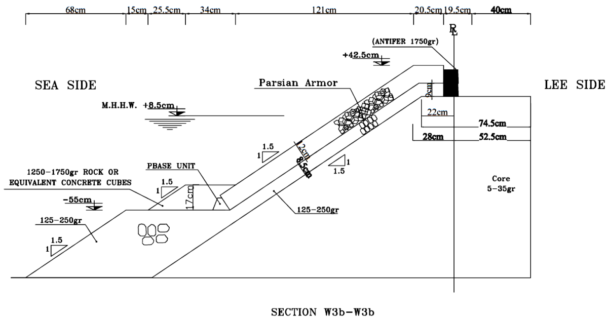
شکل ۴- ابعاد مقطع مدل آزمایشگاهی موج شکن بندر پارسیان
