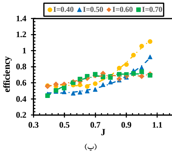
شکل ۱۳- منحنی ضرایب هیدرودینامیکی و بازده پروانه با قطر ۰/۱۴۰ در نسبت‌های مغروقیّت مختلف
