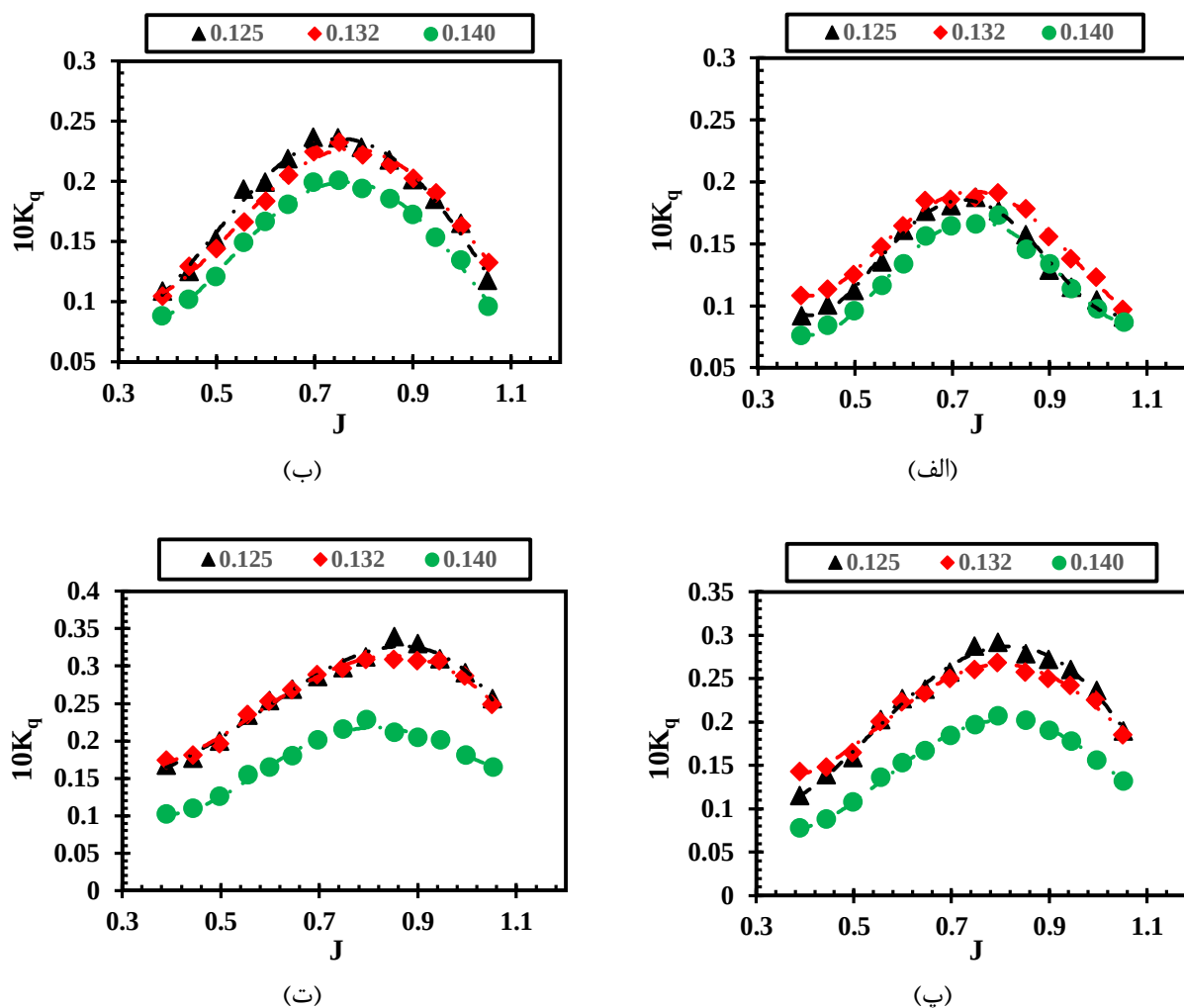
شکل ۹- منحنی ضریب گشتاور سه پروانه در نسبت‌های مغروقیّت (الف) ۰/۴۰ (ب) ۰/۵۰ (پ) ۰/۶۰ (ت) ۰/۷۰
