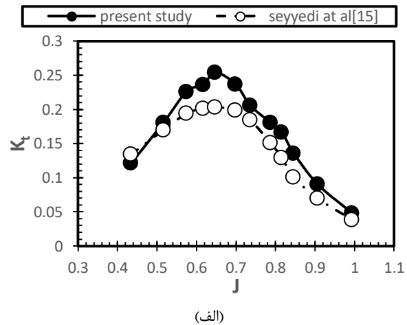
شکل ۷- مقایسه ضرایب (الف) تراست (ب) گشتاور با نتایج سیدی و همکاران (۲۰۱۹)
