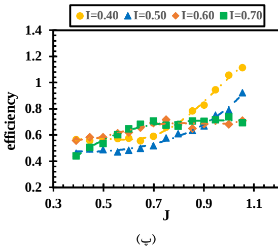
شکل ۱۳- منحنی ضرایب هیدرودینامیکی و بازده پروانه با قطر ۰/۱۴۰ در نسبت‌های مغروقیت مختلف
