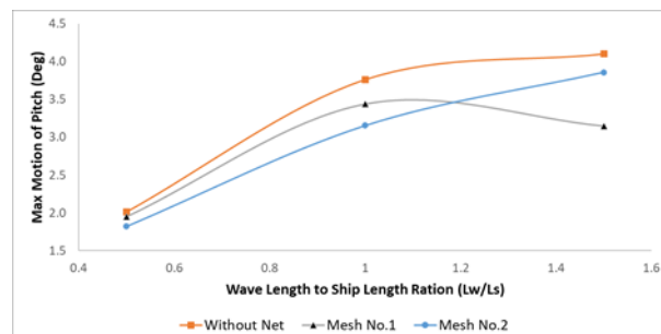
شکل ۱۸- مقایسه ماکزیمم حرکت پیچ مدل، مابین تور با مش ۱ و مش ۲ با بدنه بدون تور
