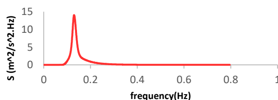
شکل ۷- توزیع طیف موج جانسواپ ۹
