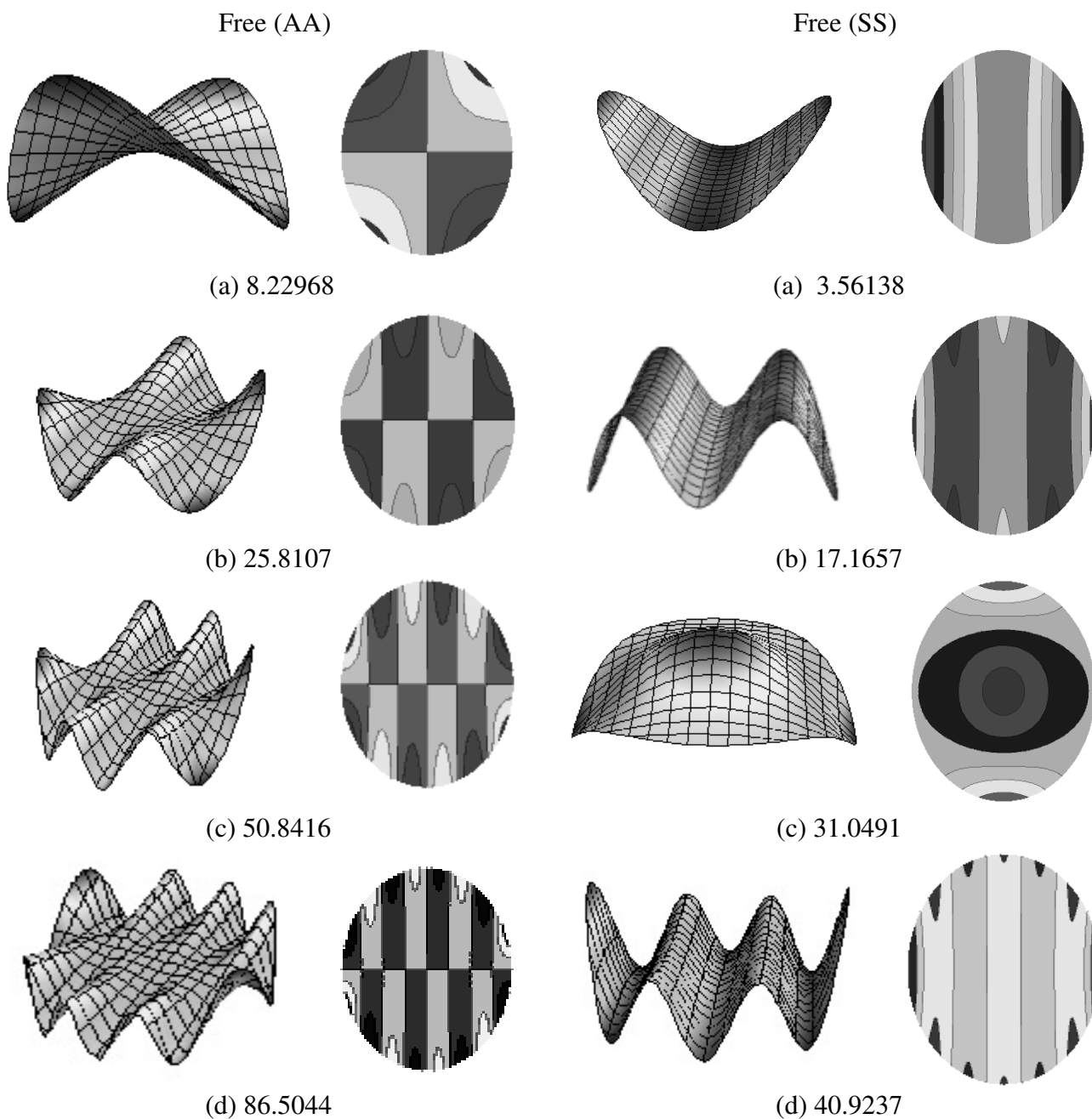
شکل ۴-الف- شکل مدهای متقارن- متقارن و پادمتقارن- پادمتقارن یک ورق بیضوی FGM با لبه آزاد
