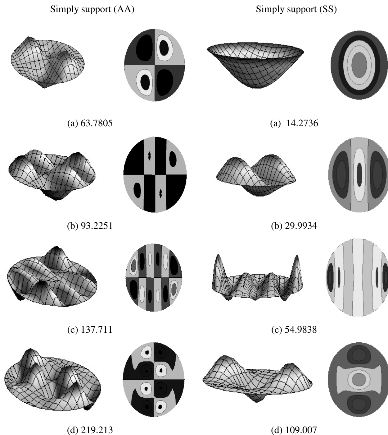
شکل ۵- شکل مودهای متقارن - متقارن و پادمتقارن - پادمتقارن یک ورق بیضوی FGM با لبه تکیه‌گاهی ساده
