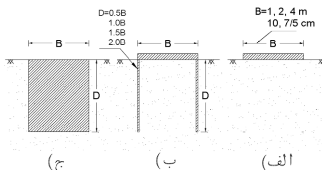
شکل ۴- جزئیات انواع مدل های پی؛ الف) سطحی، ب) لبه دار، ج) نیمه عمیق
