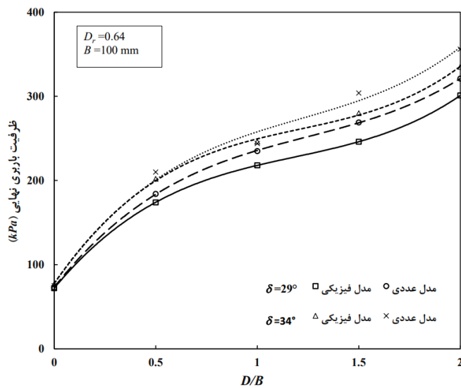
شکل ۱۶- مقایسه مقادیر ظرفیت باربری نهایی مدل های پی بر اساس نتایج مدل سازی فیزیکی و عددی
