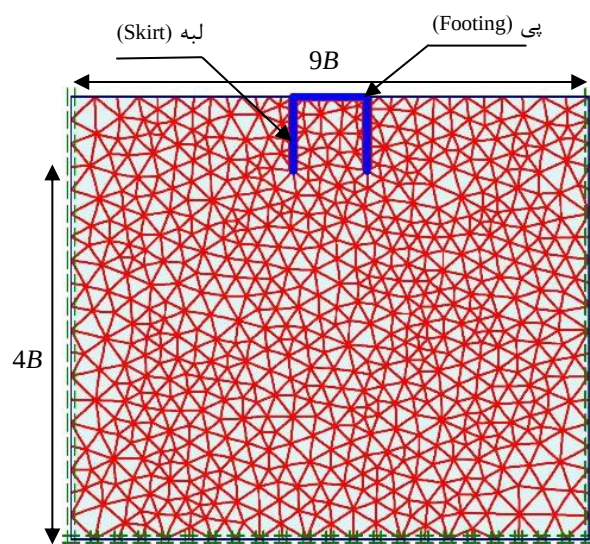
شکل ۳- ابعاد شبکه المان و شرایط مرزی مدل سازی
