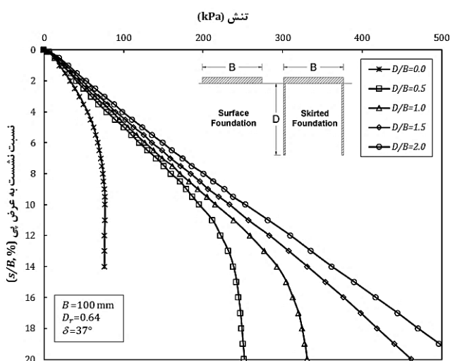
شکل ۹- پاسخ تیپ تنش- نسبت نشست پی لبه دار مدل سازی فیزیکی
