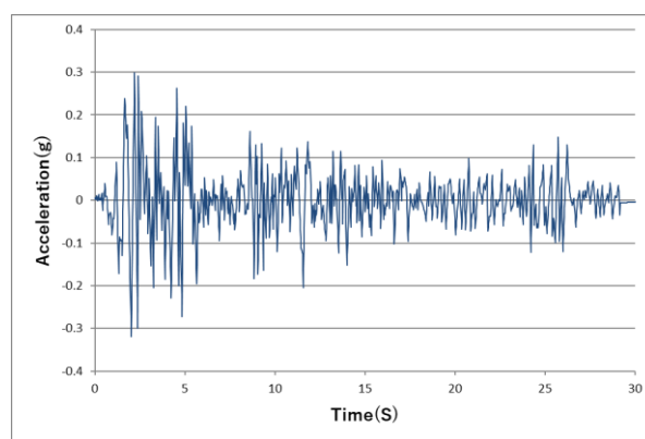
شکل ۷: شتاب نگاشت زلزله ال سنترو
