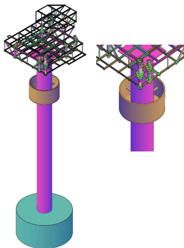
شکل ۳: شماتیک مخزن خارجی TLD بر روی تک پایه
