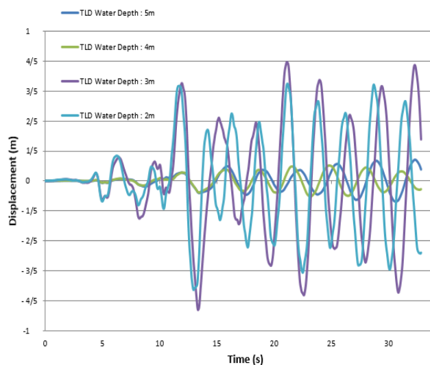
شکل ۹: مقایسه جابجایی تک پایه برای عمقهای متفاوت آب در تانک TLD در زلزله طیس
