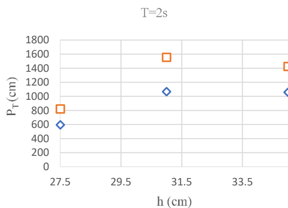
شکل ۱۰ ج: تغییرات فشار خروجی در برابر عمق آب برای دوره تناوب ۲s
