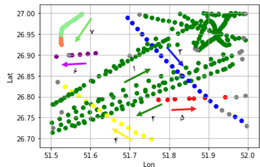
شکل ۲۲ - نتیجه خوشه‌بندی برای ۵۰۰ داده
