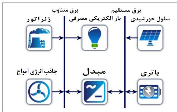
شکل ۹- شماتیک سیستم هیبریدی برای تأمین برق منطقه کمبل سلیمان
