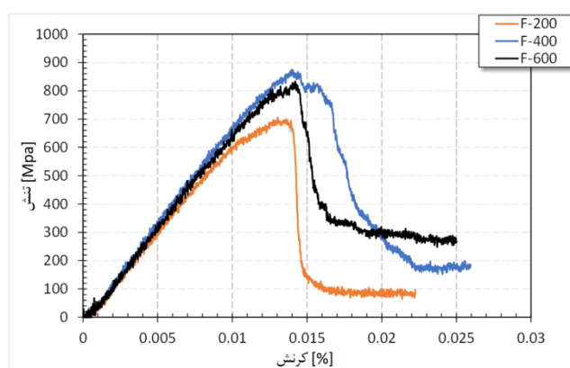
شکل ۹- نمودار تنش-کرنش حاصل از تست خمشی سه نقطه‌ای نمونه‌های شامل لایه‌های با دانسیته سطحی، ۲۰۰، ۴۰۰ و ۶۰۰ گرم بر متر مربع
