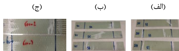
شکل ۶- شکل هندسی قطعات پس از انجام آزمون خمشی سه نقطه‌ای، قطعات ساخته شده از الیاف با دانسیته (الف) ۲۰۰ گرم بر متر مربع، (ب) ۴۰۰ گرم بر متر مربع، (ج) ۶۰۰ گرم بر متر مربع
