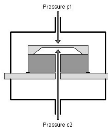
شکل (۳) منطق اندازه‌گیری توسط حسگر فشار تفاضلی
