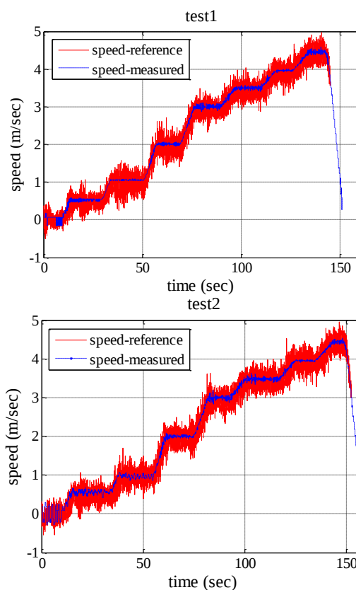
شکل (۶) خروجی سرعت مرجع و سرعت اندازه‌گیری شده توسط حسگر سرعت پیشنهادی در تست‌های ۱ و ۲.
