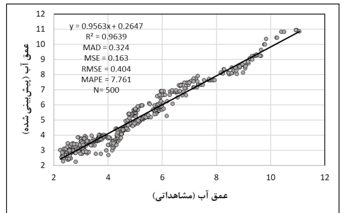
شکل ۷- نمودار پراکندگی مقادیر عمق آب مشاهداتی در محدوده نقاط کنترلی (۵۰۰ نقطه) در مقابل عمق آب برآورد شده با استفاده از تصاویر Landsat-OLI و رابطه رگرسیونی شماره ۳ جدول ۱- جدول تحلیل واریانس مربوط به رابطه رگرسیونی برازش داده شده جهت برآورد عمق آب
