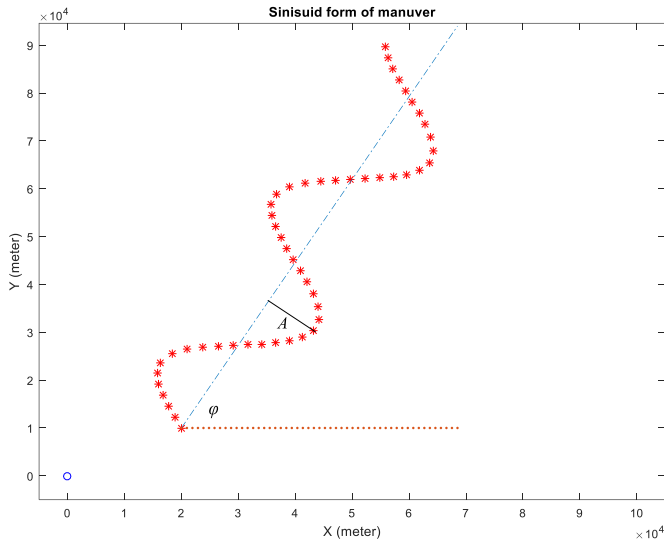
شکل ۲: نمونه ای از حرکت تهدید با مانور زیگزگی سینوسی (با پارامترهای \varphi=60 Deg, \omega=1.57e-4 , A=1000 y_T(0) = 10000 و x_T(0) = 20000 )
